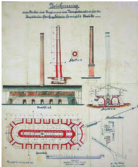
1900 výkres cihlářské pece
